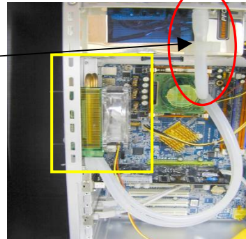
Plastikhalterung
