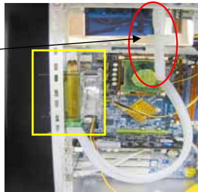
SilentStream® 升級版 快速版安裝完成圖 （冷排置於機殼內，安裝快速完成）
