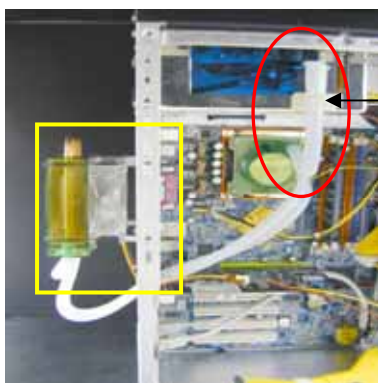
SilentStream® 升級版 專業版安裝完成圖 （冷排置於機殼外，散熱效果最佳）
