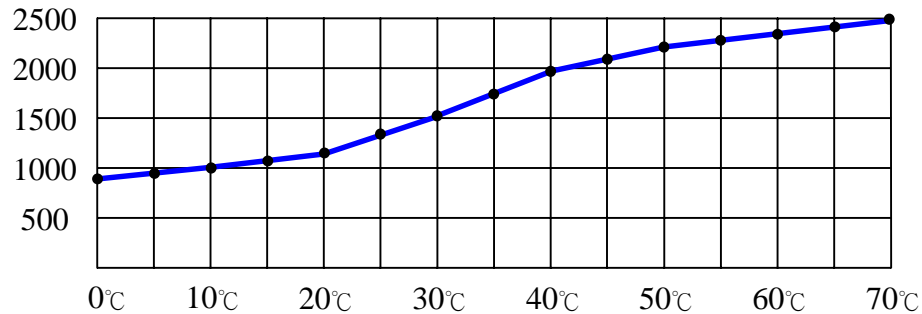
R.P.M FAN SPEED CURVE: 800RPM~2,500RPM ± 100 R.P.M
